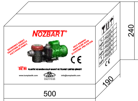
Teknik Ölçüler (mm) / Dimensions (mm)
