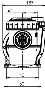
Teknik Ölçüler (mm) / Dimensions (mm)
