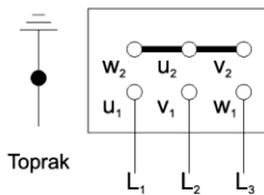
Y-Bağlantı Üç Faz (b)
